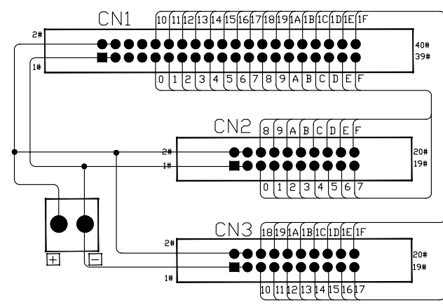
接線圖 / Connection Diagram
