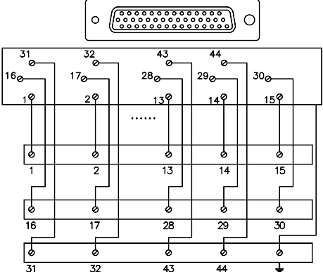
接線圖 / Connection Diagram
