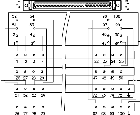
接線圖 / Connection Diagram
