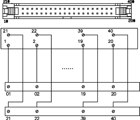
接線圖 / Connection Diagram
