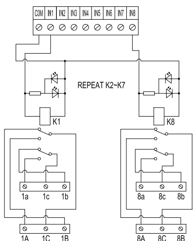
接線圖 / Connection Diagram
