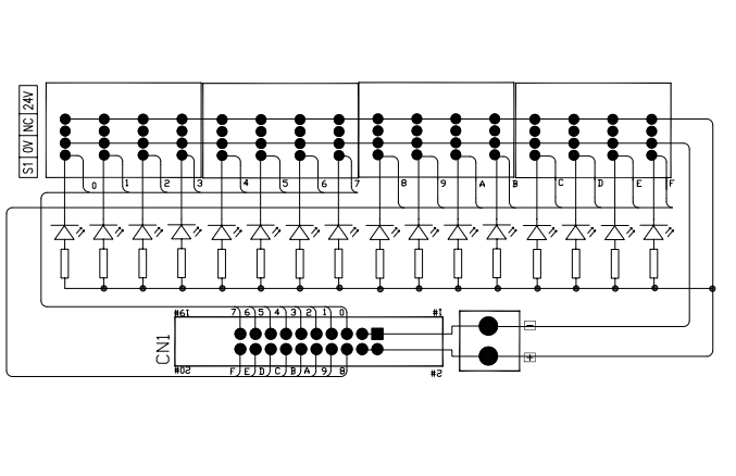
接線圖 / Connection Diagram
