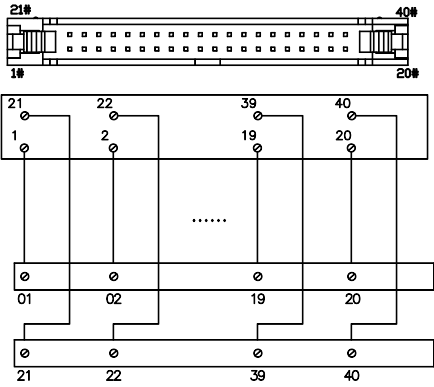
接線圖 / Connection Diagram
