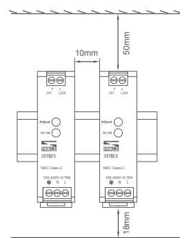
電源安裝空間建議距離
